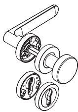
AVUS Schraub Wechselgarnitur Ausführungen: PZ, RZ mit Knopf R2
